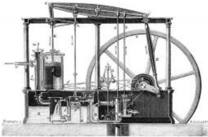
Fig. 26. — Mécanisme à balancier de Watt.
